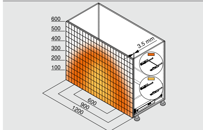
560H 的示例 – 30 kg, 标称长度 NL 500 mm, 四面抽屉, 配有同步装置
