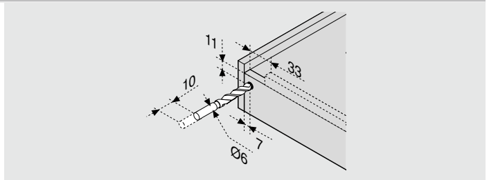
使用钻模 T65.1000.02
