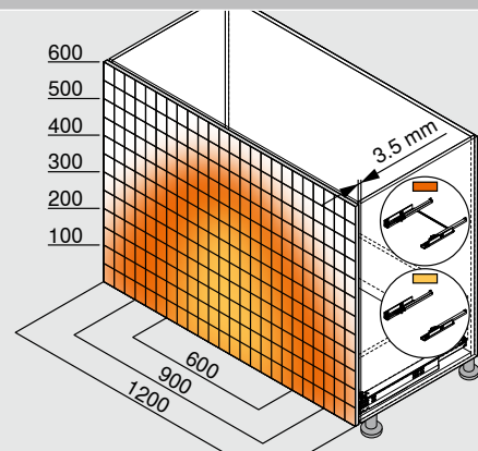
以550F 为例 – 30 kg, 导轨长度 NL 500 mm, 四面抽屉, 配有同步装置
