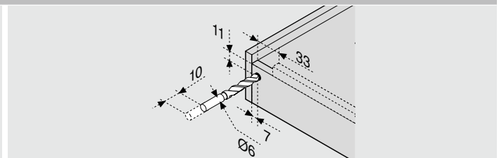
使用钻模 T65.1000.02
