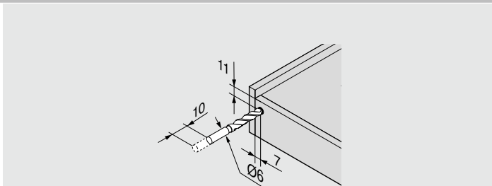
使用钻模 T65.1000.02
