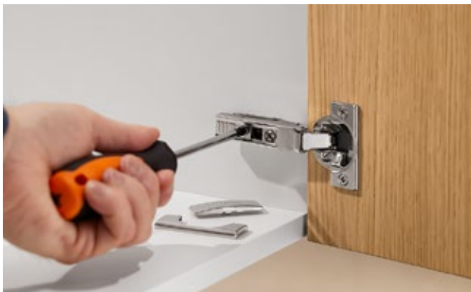
三维面板调节, 通过偏心螺丝进行无级深度调节
